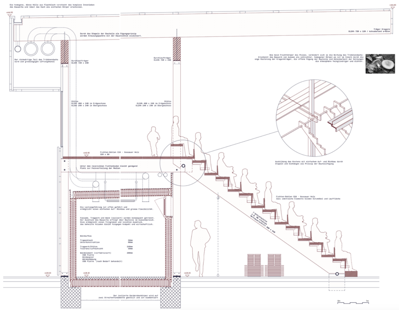
Fassadenschnitt
