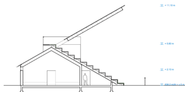
Schnitt 2
