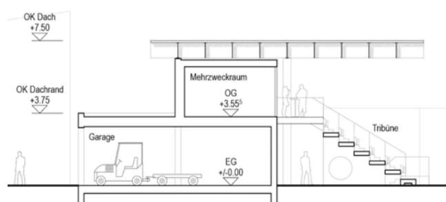
Schnitt 1
