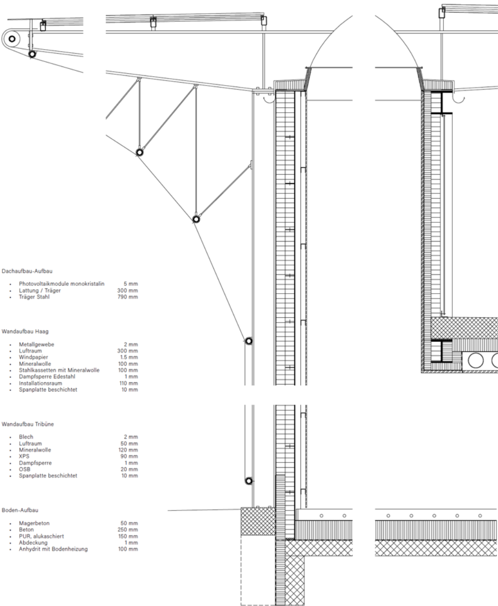
Fassadenschnitt
