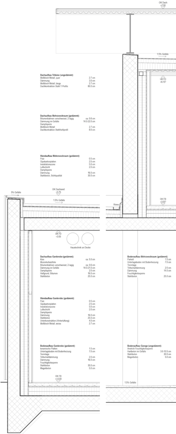
Fassadenschnitt
