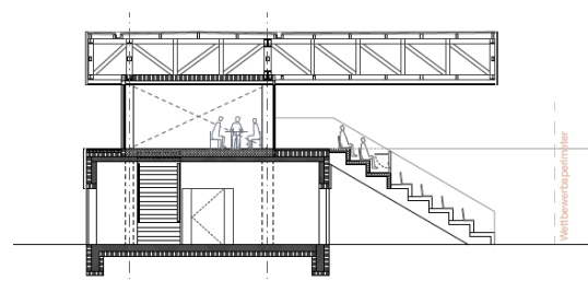
Schnitt 1
