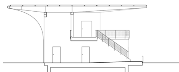
Schnitt 1
