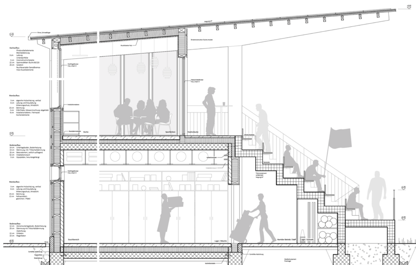
Fassadenschnitt
