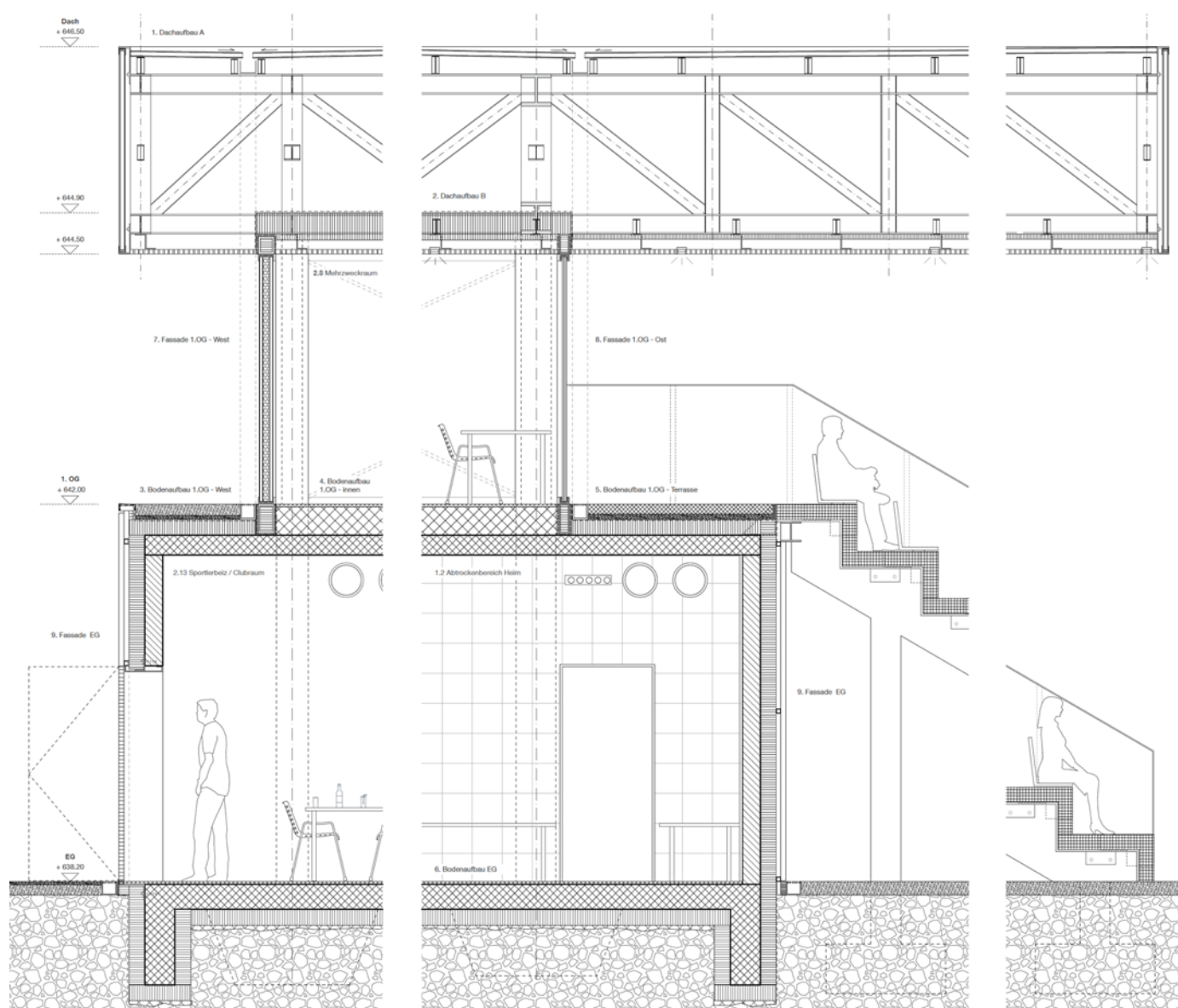
Fassadenschnitt
