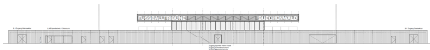
Ansicht West
