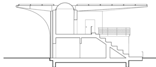
Schnitt 2
