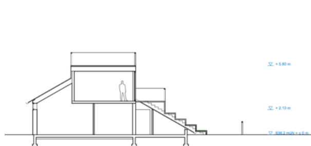
Schnitt 1
