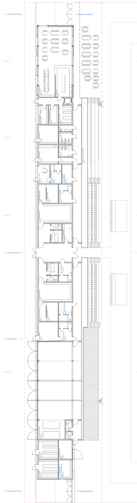
Erdgeschoss
