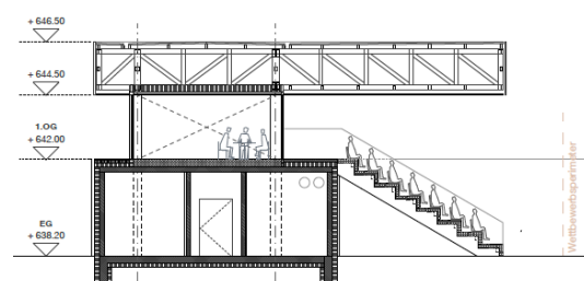
Schnitt 2
